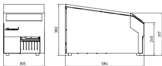
ES-M zonder scherm
